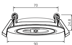
TILT TRIM Ø80
